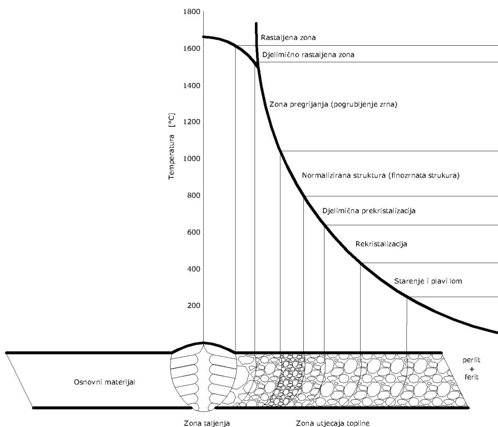
Slika 5. Utjecaj unosa topline na strukturu zavaa [3]
