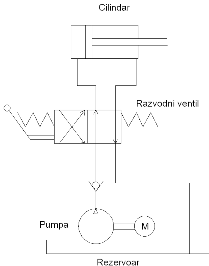
Slika 12. Hidraulička shema
