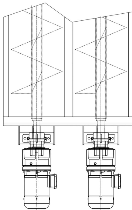
Slika 22. Prikaz pogona i krajnjih radijalno-aksijalnih ležaja
