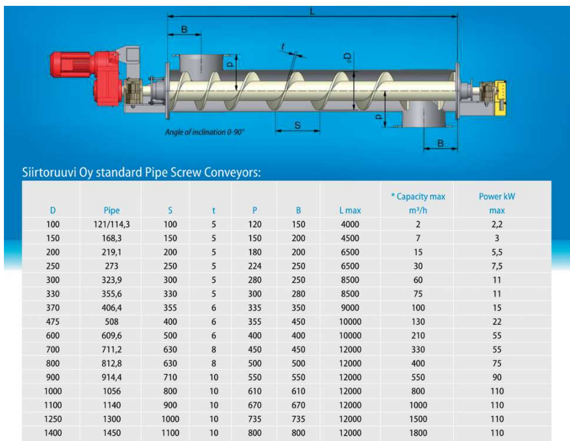
Tablica 2. Vrijednosti raznih izvedbi velikih Siirtoroovi konvejera sa cijevi [5]
