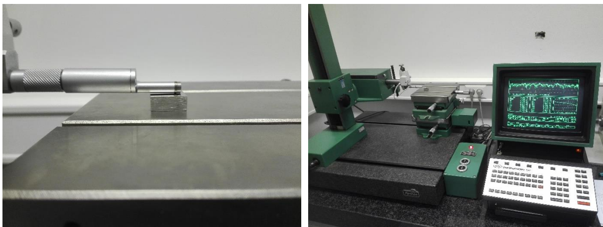
Slika 28. a) Pomicanje ticala po ispitnom uzorku, b) uređaj za mjerenje hrapavosti
