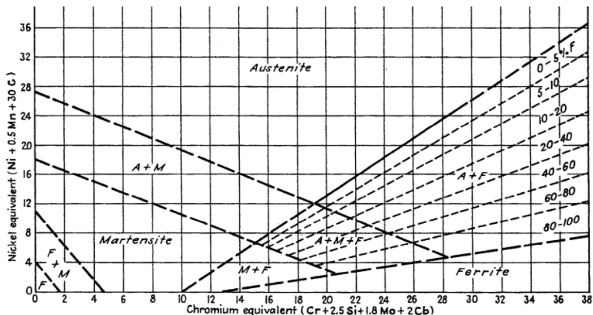
Slika 1. Schöfflerov dijagram struktura nehrđajućih čelika [3]
