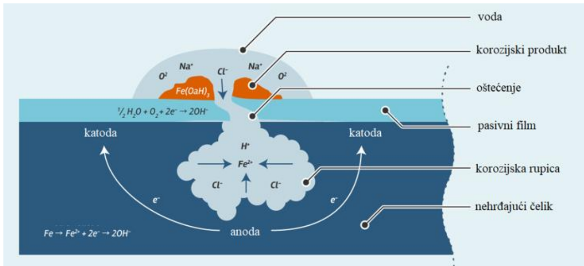
Slika 14. Shematski prikaz rupičaste korozije [19]
