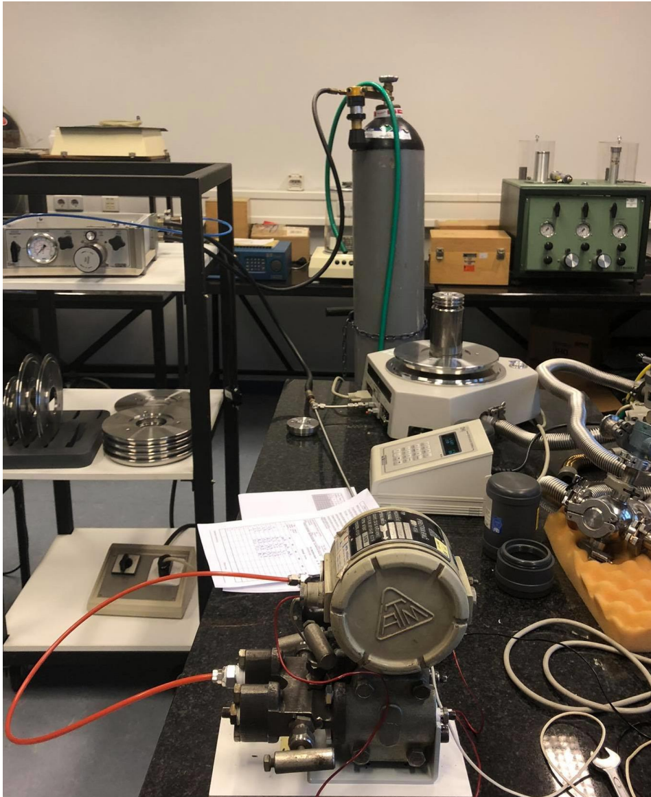
Slika 18. Umjeravanje tlačnom vagom TLVAG 09
