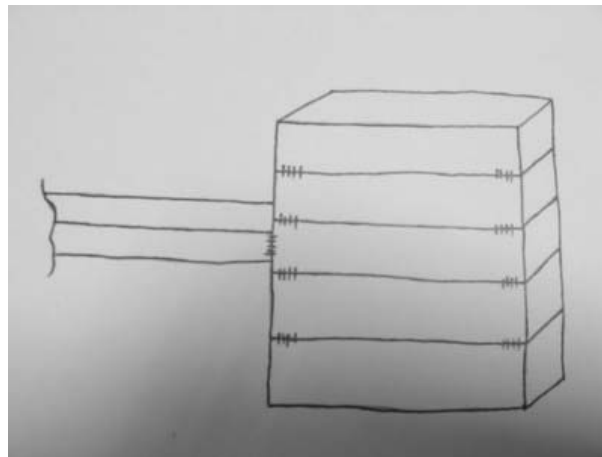
Slika 2. Složeni i osigurani slojevi kao priprema za kovačko zavarivanje
