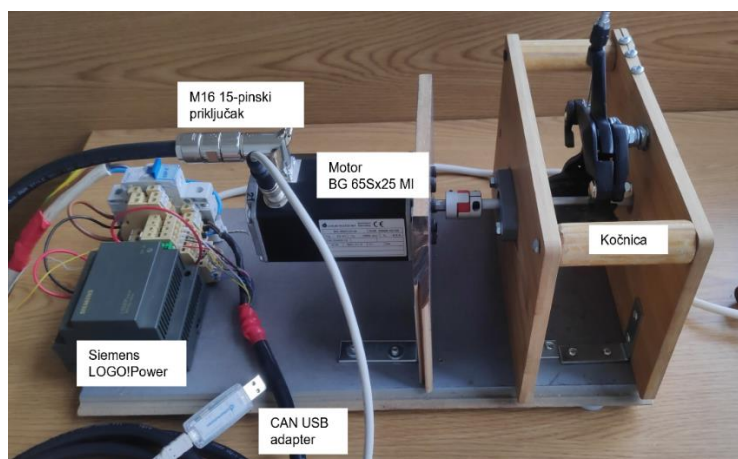
Slika 35. Eksperimentalni postav
