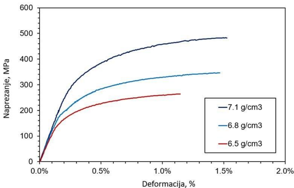
Slika 4 Naprezanje u ovisnosti o deformaciji za različite gustoće sinteriranog čelika
