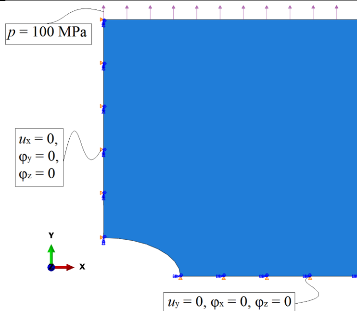
Slika 15 Rubni uvjeti i opterećenje pore eliptičnog oblika
