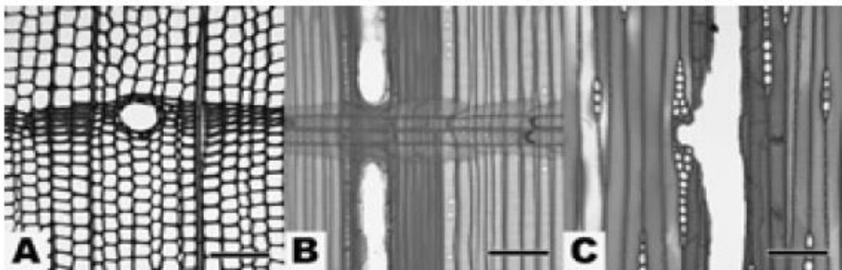
Slika 16. Smolni kanal u aksijalnom (A), radijalnom (B) i tangencijalnom presjeku (C) [6]
