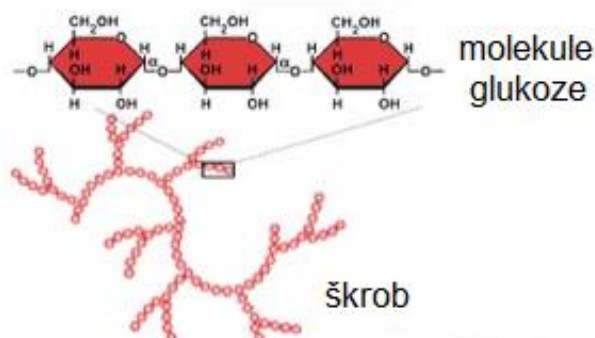
Slika 12. Struktura škroba [5]
