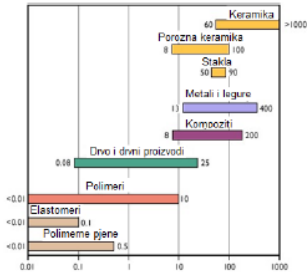
Slika 18. Vrijednosti modula elastičnosti za različite tehničke materijale u GPa [7]
