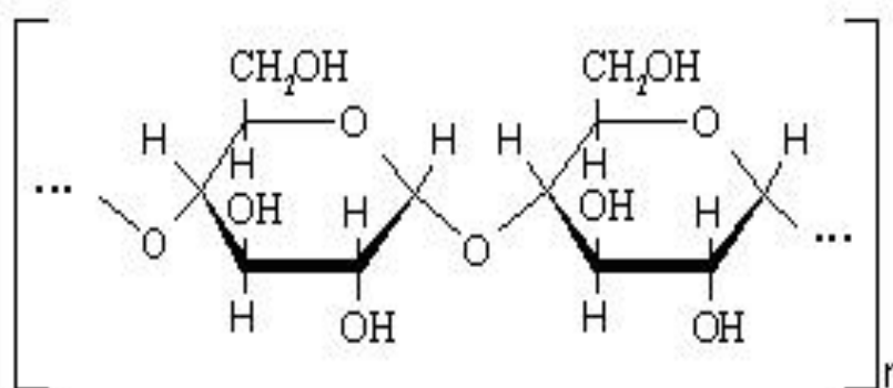
Slika 8. Struktura celuloze [6]
