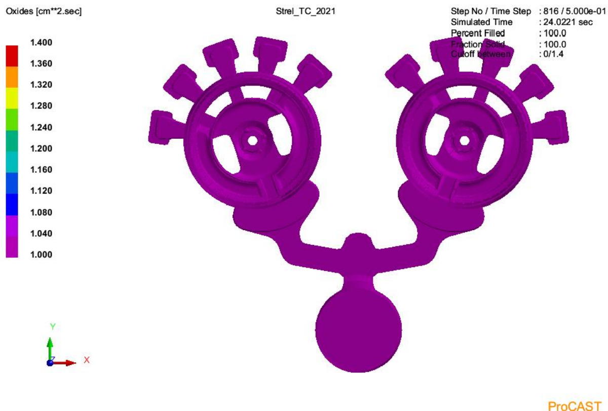
Slika 46. Zarobljeni oksidi 2.
