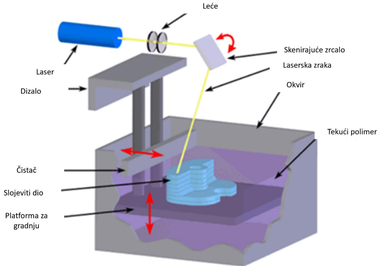
Slika 4. Stereolitografija [5]
