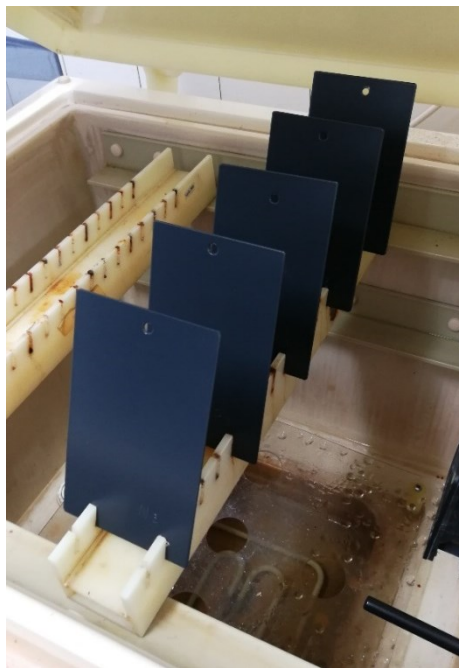
Slika 38. Uzorci u vlažnoj komori neposredno nakon početka ispitivanja
