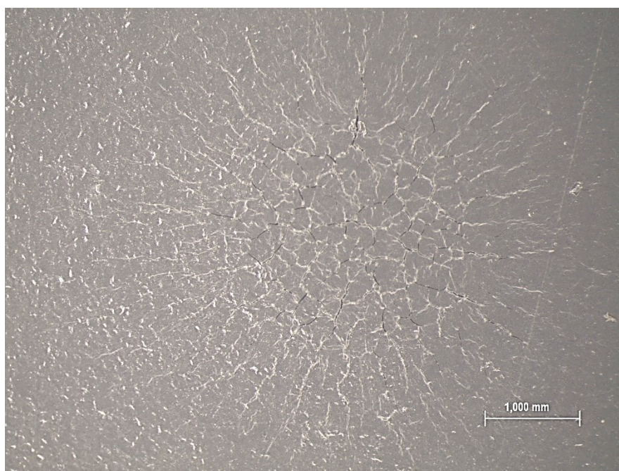
Slika 63. Uzorak P3 - ne zadovoljava; visina s koje je pušten uteg pri kojoj prevlaka nije zadržala svoja svojstva kao ni mikro i makro konzistentnost iznosi 10 cm
