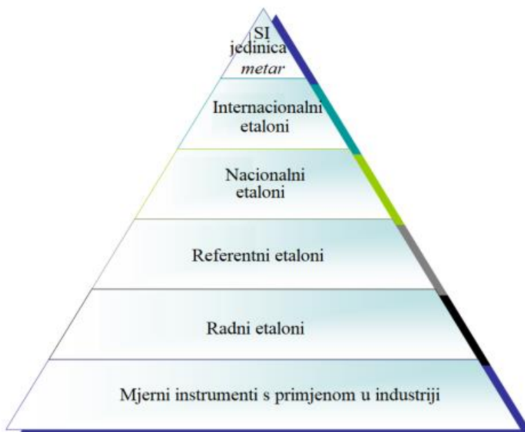
Slika 1. Piramida sljedivosti [2]
