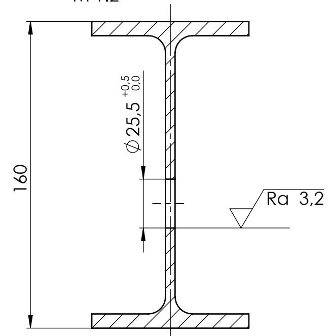
Presjek A-A M 1:2
