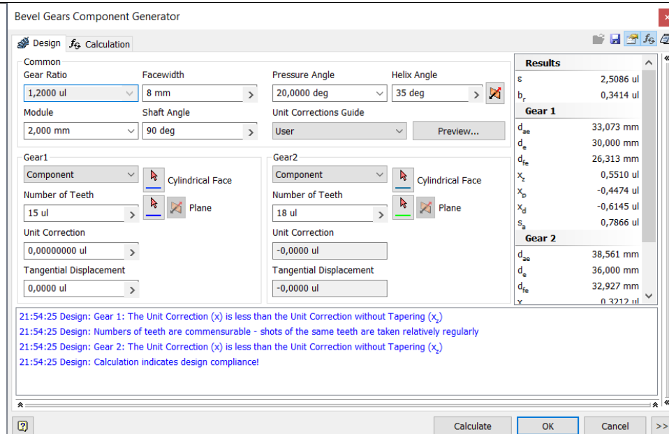
Slika 38 Proračun stožnika #2
