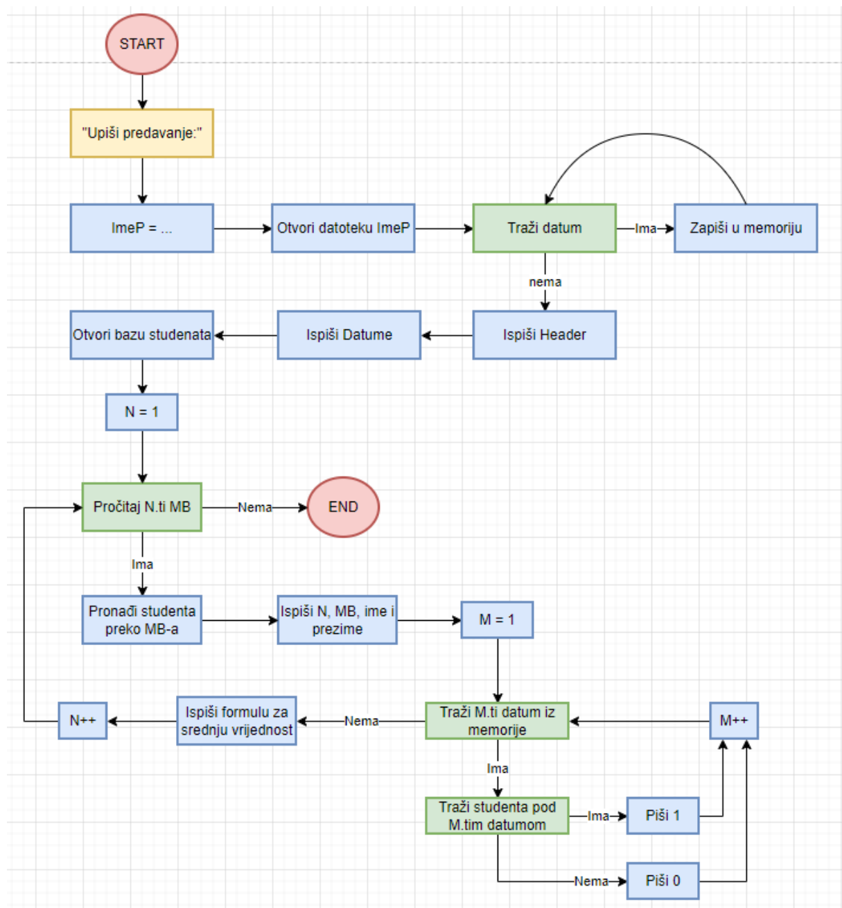
Slika 18. Naredba "Tablica"
