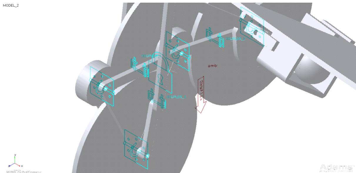
Slika 26. Kinematička ograničenja nosača i zupčanika mehanizma pokretnog krila II
