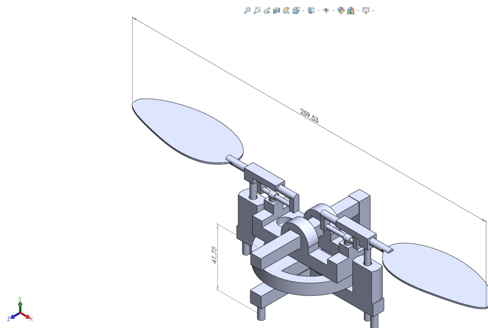
Slika 39. Model za tiskanje mehanizma pokretnog krila I
