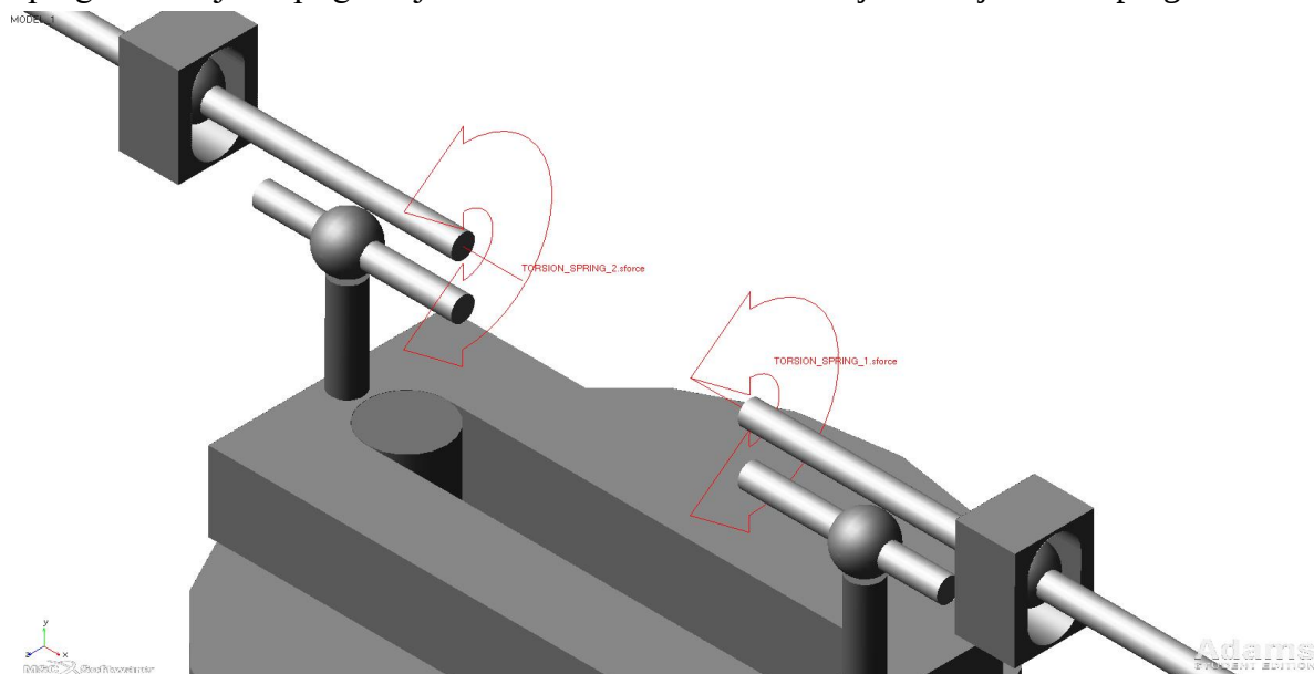
Slika 24. Položaj opruga na mehanizmu pokretnog krila I
