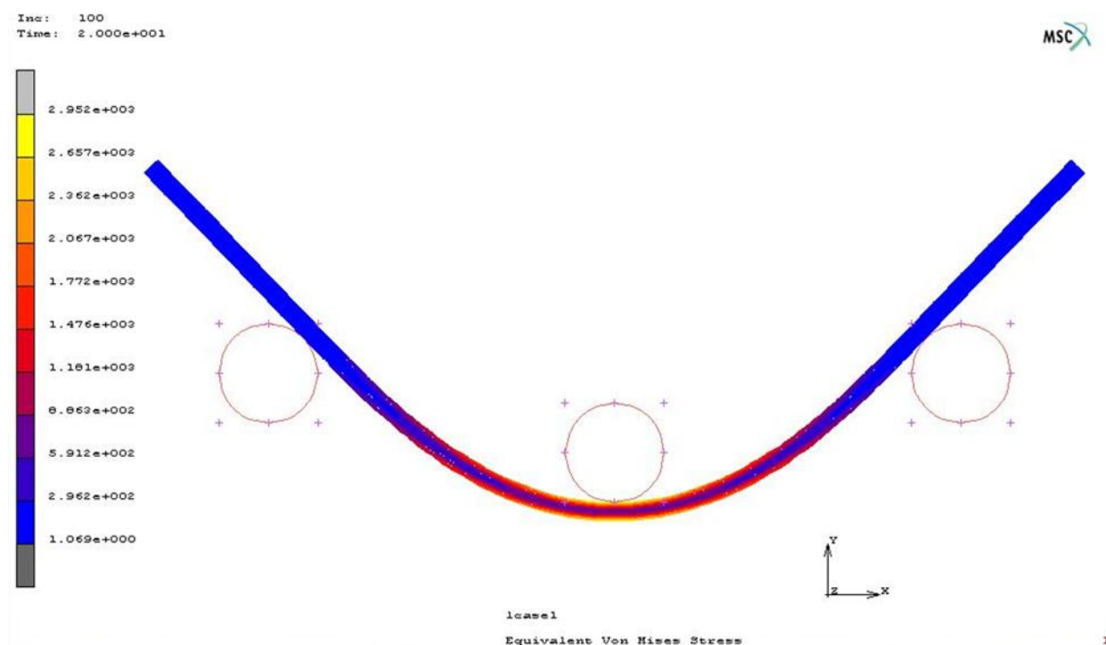
Slika 23. Raspored naprezanja za aluminijski lim AlMg3
