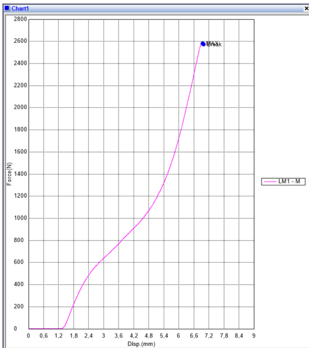
Slika 5.13 Dijagram "sila-progib" za epruvetu LM1--M
