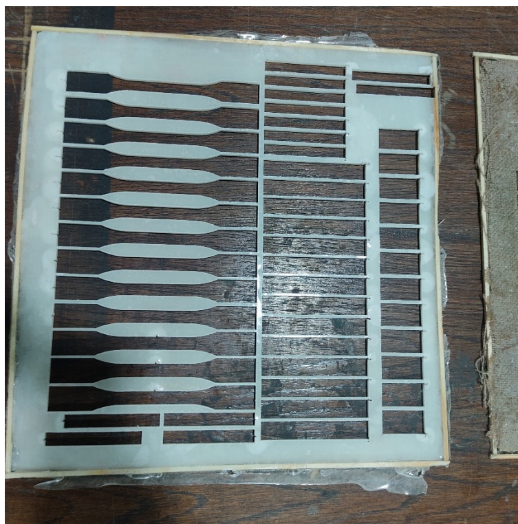
Slika 4.17 Epruvete za ispitivanje mehaničkih svojstva
