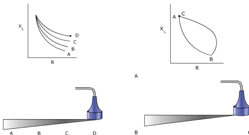
Slika 48: Mjerenje debljine [4]
