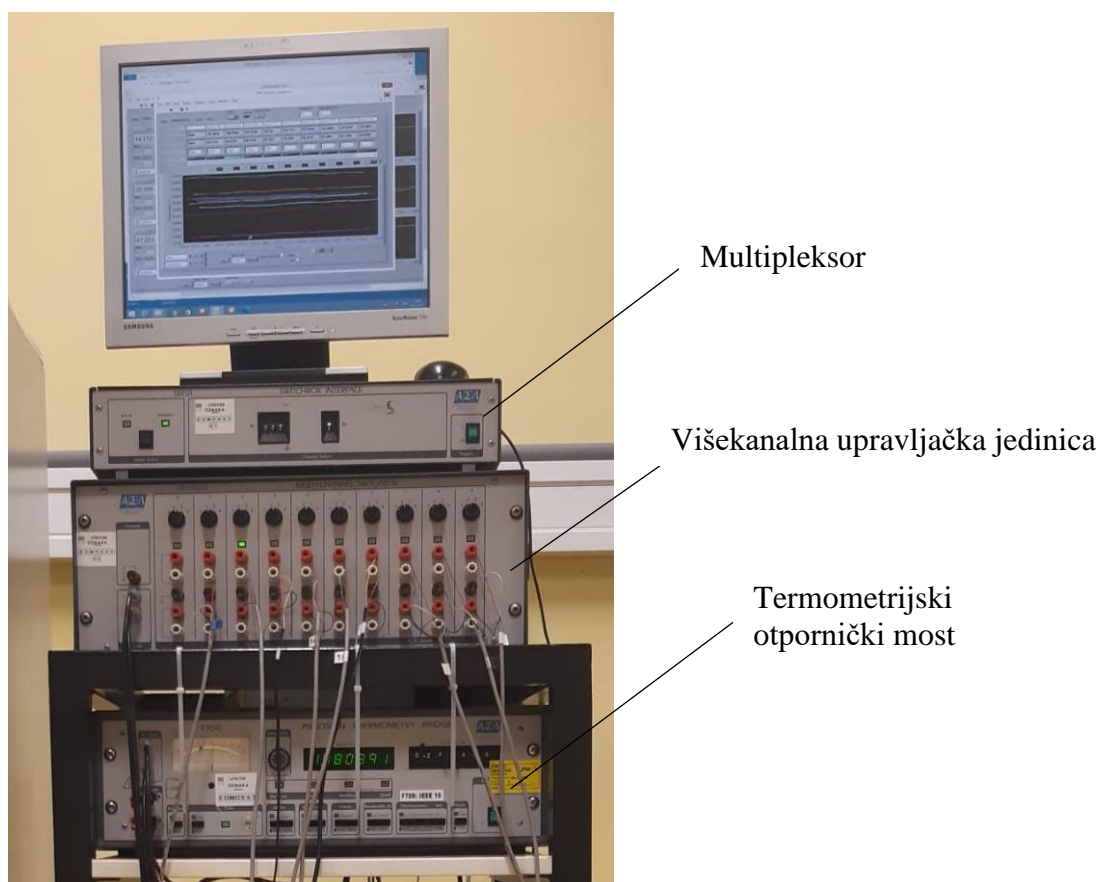
Slika 4. Mjerna postaja
