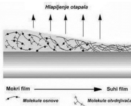
Slika 14. Dvokomponentno sušenje [4]
