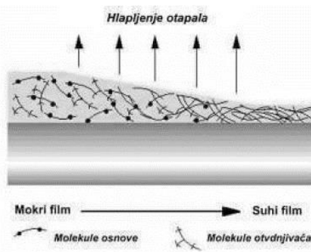
Slika 14. Dvokomponentno sušenje [4]
