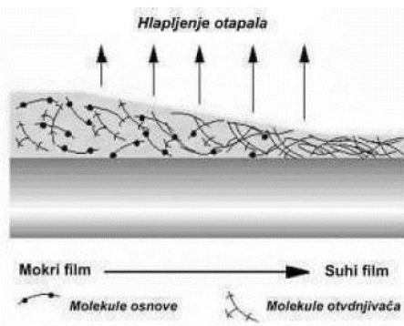
Slika 14. Dvokomponentno sušenje [4]
