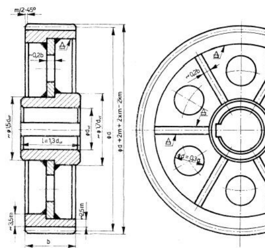
Slika 9. Zavareni zupčanik 2 [2].
