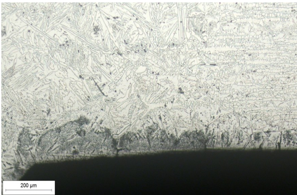
Slika 44. Mikrostruktura ZUT-a, desno, u korijenu zavora, snimljena pri povećanju 100×
