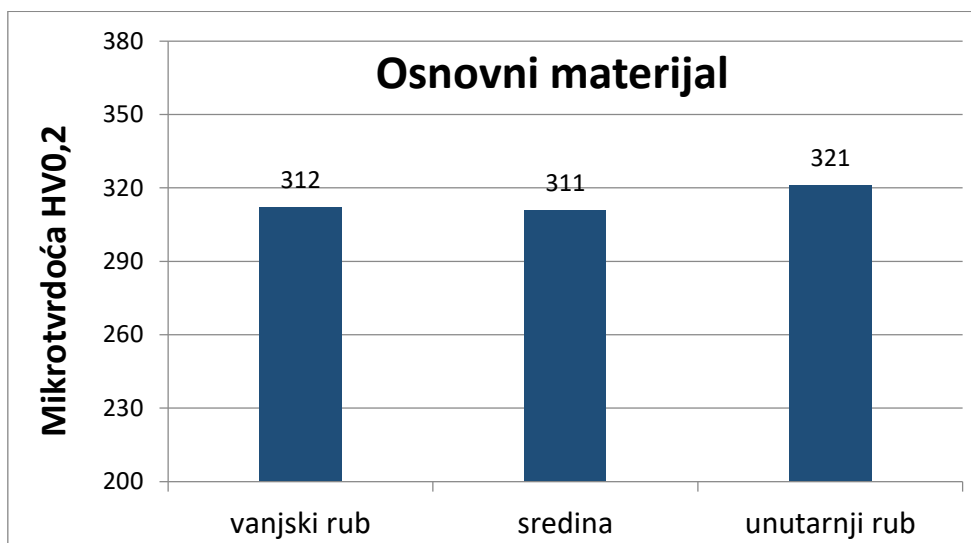
Slika 52. Mikrotvrdoća HV0,2 u osnovnom materijalu
