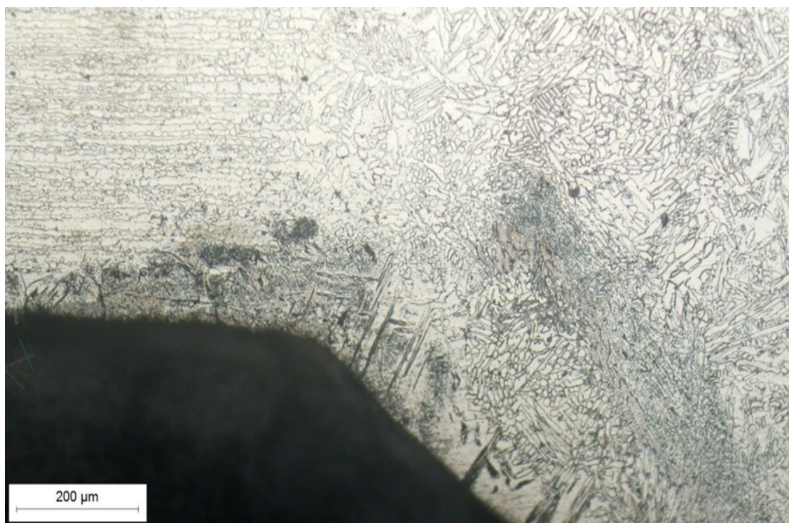
Slika 43. Mikrostruktura ZUT-a, lijevo, u korijenu zavora, snimljena pri povećanju 100×
