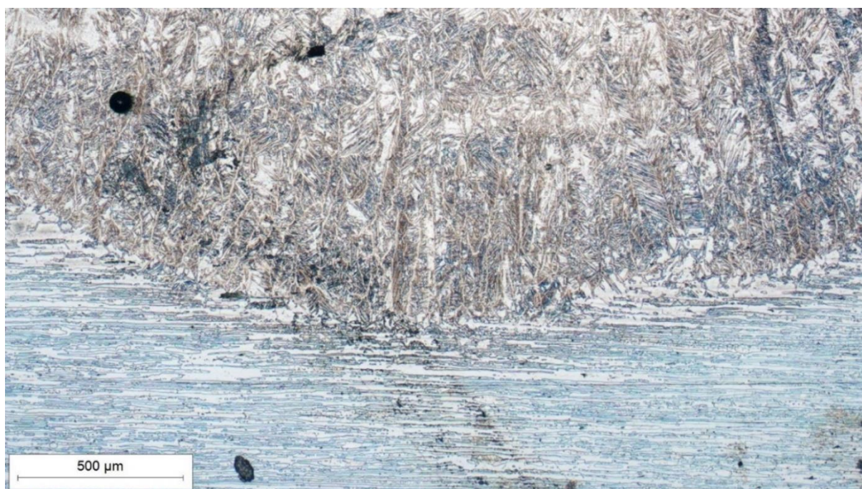
Slika 44. Mikrostruktura korijena navara uzorka 2B uz povećanje 50x
