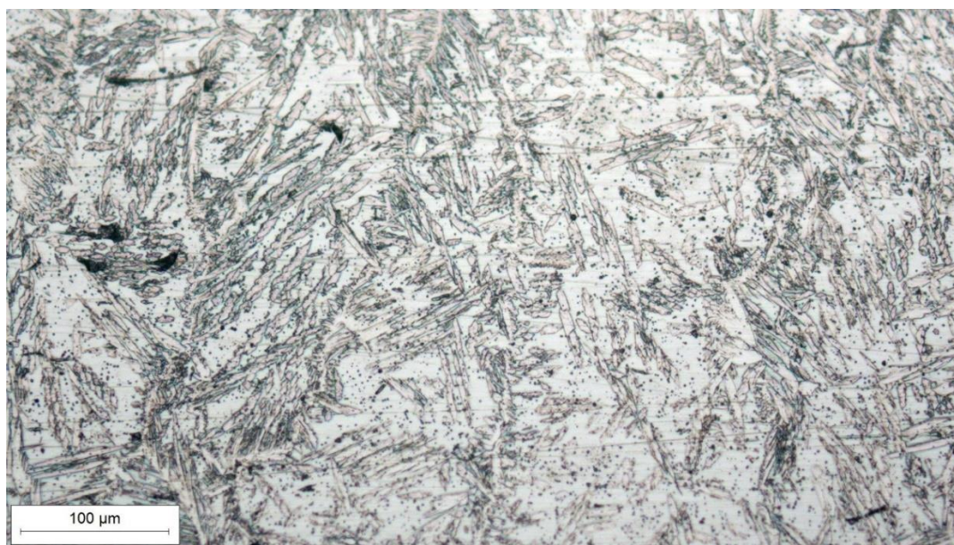
Slika 39. Mikrostruktura navara uzorka 2A uz povećanje 200x
