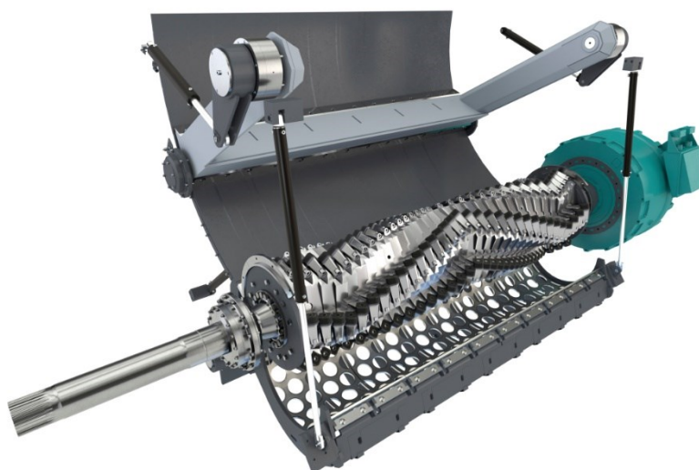
Slika 1. Jednoosovinska rezalice tvrtke Vecoplan [3]
