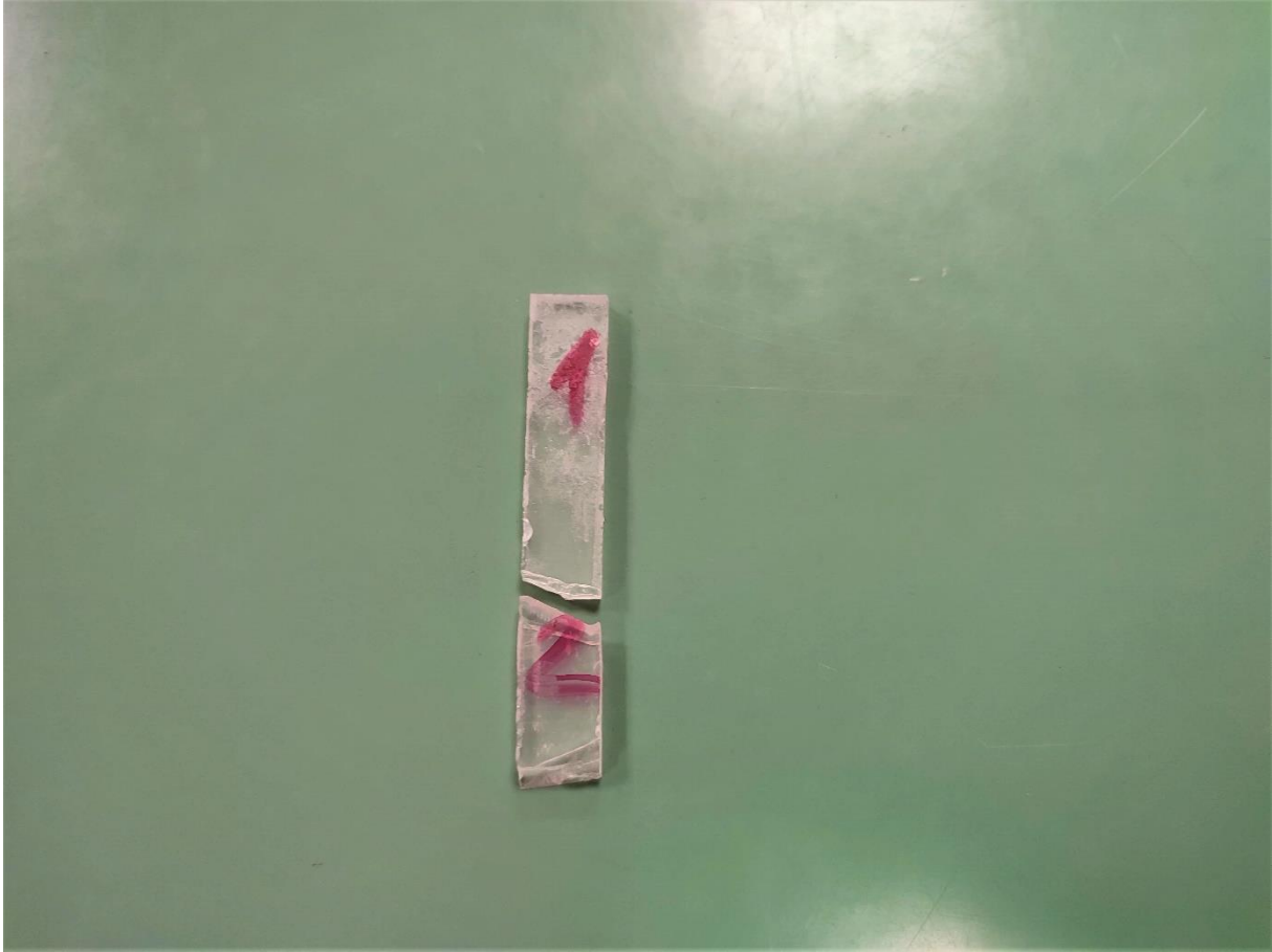
Slika 27. Slomljena epruveta nakon ispitivanja na Charpyjevom batu
