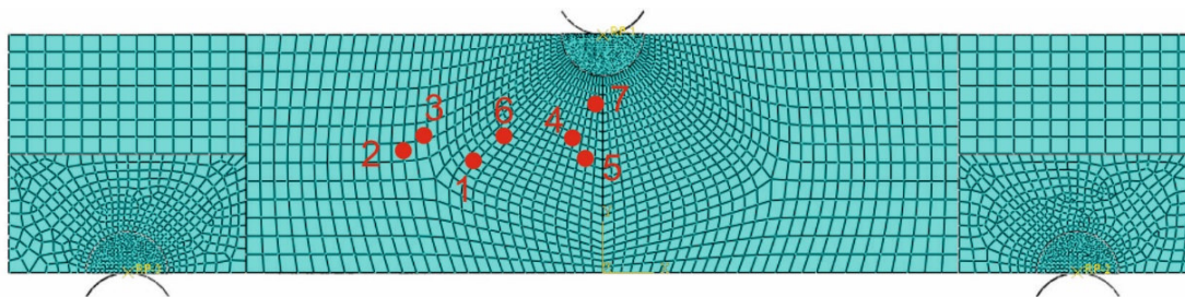
Slika 17. SEB epruveta prikaz pozicija tenzometarskih traka
