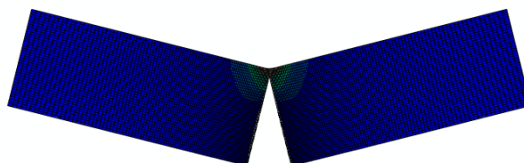
Slika 24. SEB epruveta s pukotinom na sredini: a) za početnu duljinu pukotine, b) za 60 % duljine pukotine, c) za 80 % duljine pukotine i d) 90% duljine pukotine
