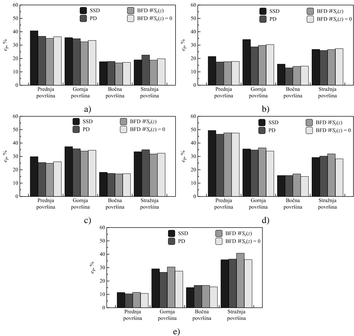
Slika 42. Srednje pogreške koeficijenta tlaka e_p izračunate računalnom simulacijom strujanja inženjerskog AGS-a oko modela zgrade koristeći modele u kojima strujanja uzrokuju smična sila (SSD), sila gradijenta tlaka (PD) i dodatna masena sila (BFD), uporabom: a) standardnog k-\varepsilon , b) RNG k-\varepsilon , c) realizable k-\varepsilon , d) Wilcoxovog k-\omega i e) Menterovog k-\omega SST modela turbulencije. Rezultati generirani koristeći model strujanja temeljen na dodatnoj masenoj sili dobiveni su korištenjem (BFD W_{S_x} ) i bez korištenja dodatne masene sile (BFD W_{S_x} = 0 ).
