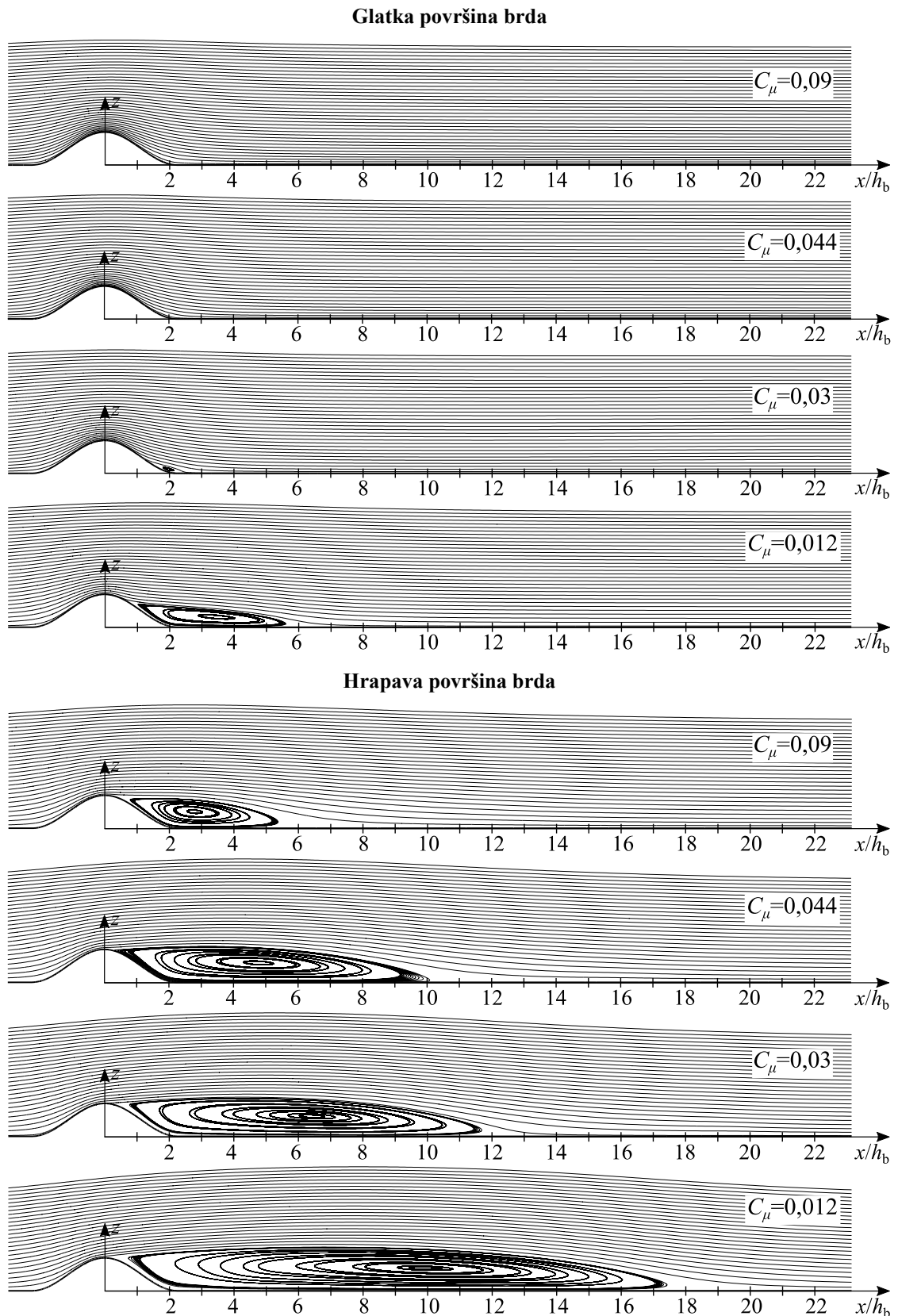
Slika 50. Usporedba strujnica generiranih računalom simulacijom strujanja inženjerskog AGS-a u kojem strujanje uzrokuje dodatna masena sila promjenjiva po visini iznad brda glatke i hrapave površine nagiba Sl_2 = 0,45 , uz korištenje različitih skupova konstanti modela turbulencije.
