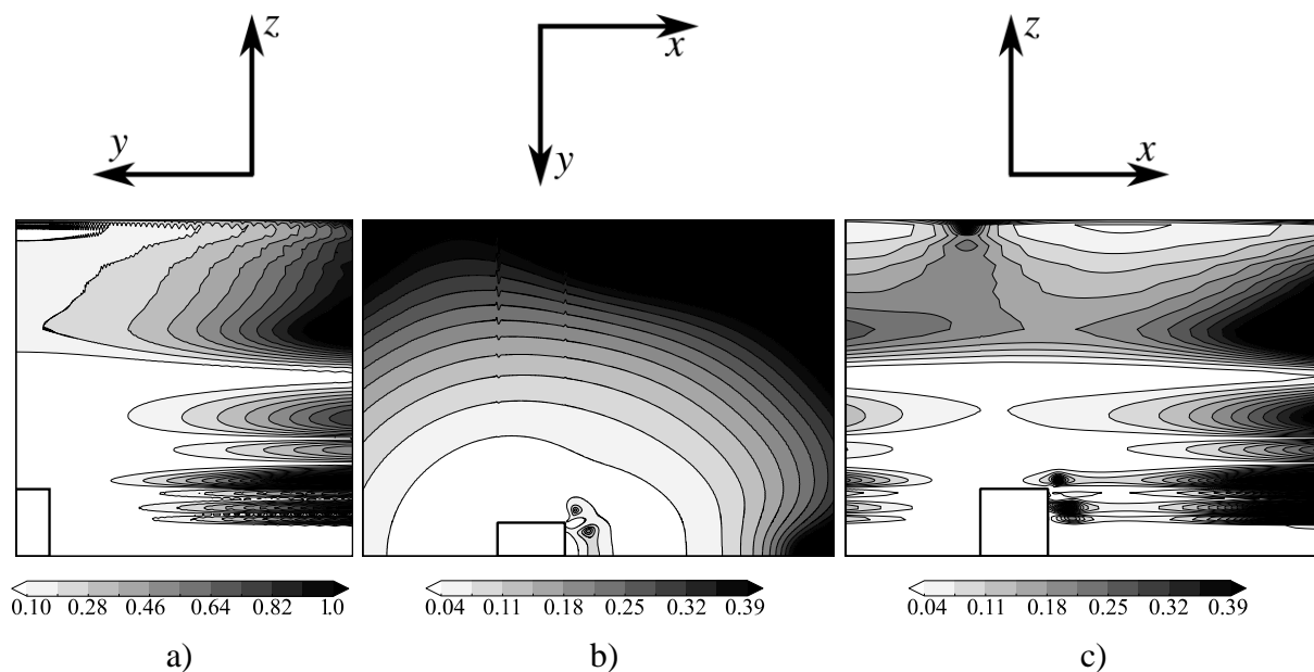
Slika 34. Skalarno polje \psi izračunato u okolini modela zgrade u ravninama a) y-z ( x = 1,1 \text{ m} ), b) x-y ( z = 0,1 \text{ m} ) i c) x-z ( y = -0,1 \text{ m} ) iz rezultata strujanja suburbanog tipa inženjerskog AGS-a oko modela zgrade.
