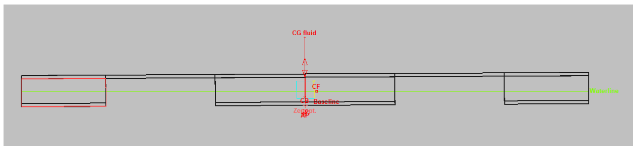
Slika 18. Prikaz naplave prostora NP1_PS iz programa MAXSURF
