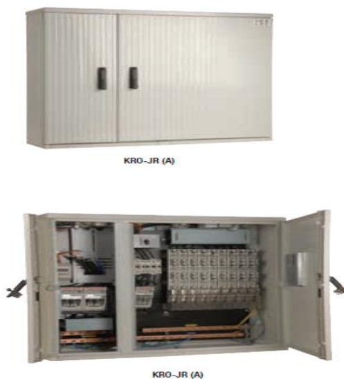
Slika 4.3. Razvodni uređaj
