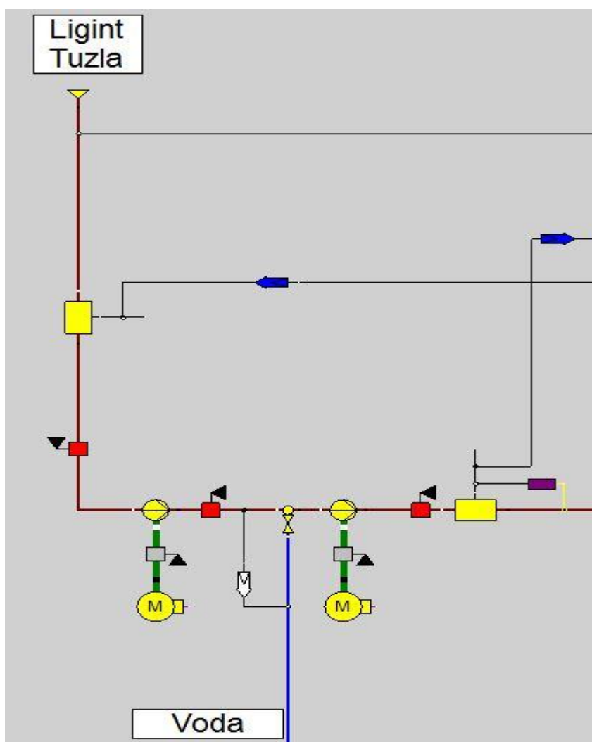
Slika 24. Prikaz miješanja ugljene prašine i vode
