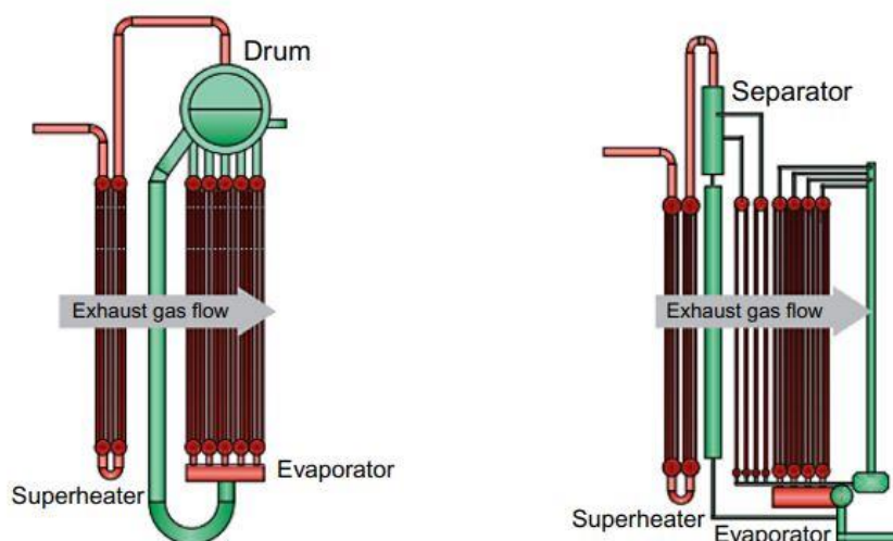
Slika 19. „Klasični“ (lijevo) i protočni (desno) generator pare [12]
