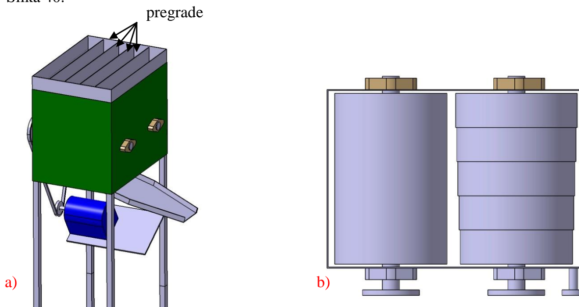
Slika 42 a) odabrana drobilica s 2 valjka b) oblik valjaka
