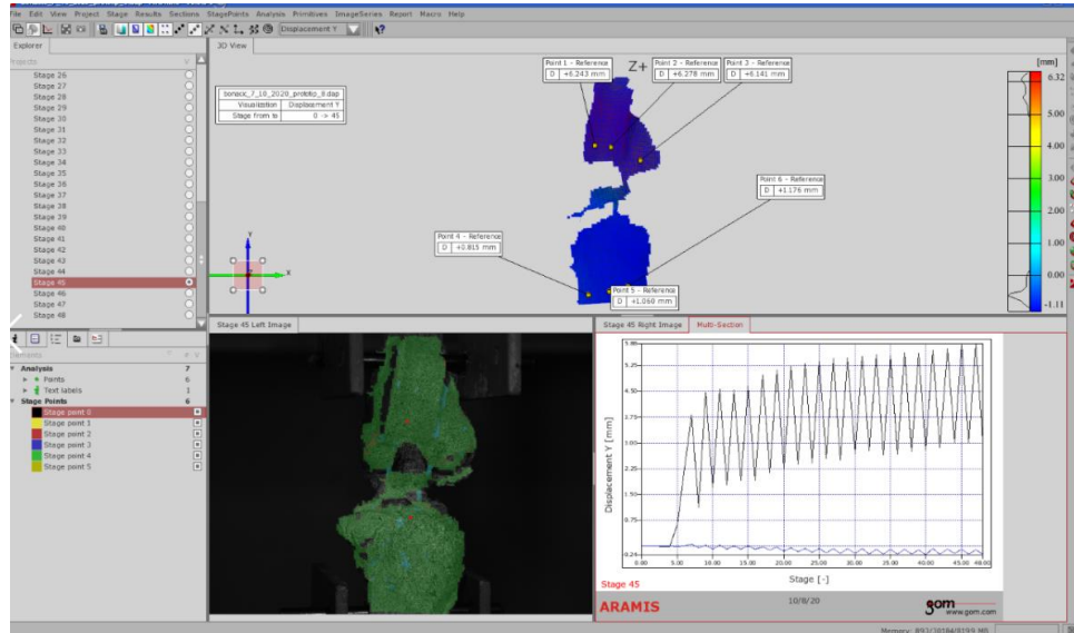
Slika 95. Prikaz upotrebljivih podataka dobivenih pomoću sustava ARAMIS, pomaci sklopa bedrena kost – prednja ukrižena sveza s ugrađenom biomehantičkom potporom – goljenica
