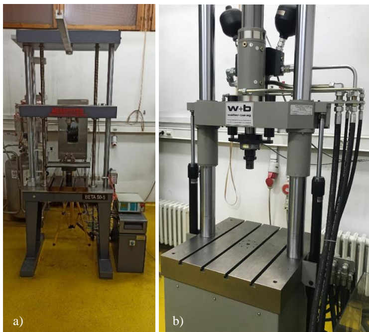
Slika 34. Prikaz a) kidalice Beta 50-5; b) umaralice LFV 50-HH
