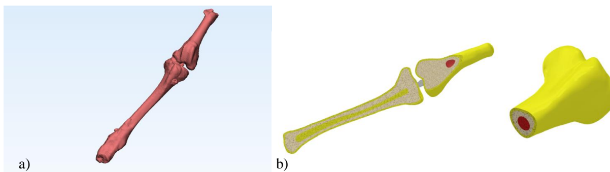
Slika 51. Prikaz a) 3D rekonstrukcija sklopa bedrena kost - prednja ukrižena sveza – goljenica iz CT skenova u programskom paketu Mimics ; b) dorađeni 3D modela sklopa bedrena kost – prednja ukrižena sveza – goljenica
