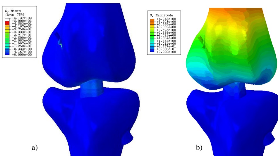
Slika 79. Model 3: raspodjela a) von Mises naprezanja; b) pomaka
