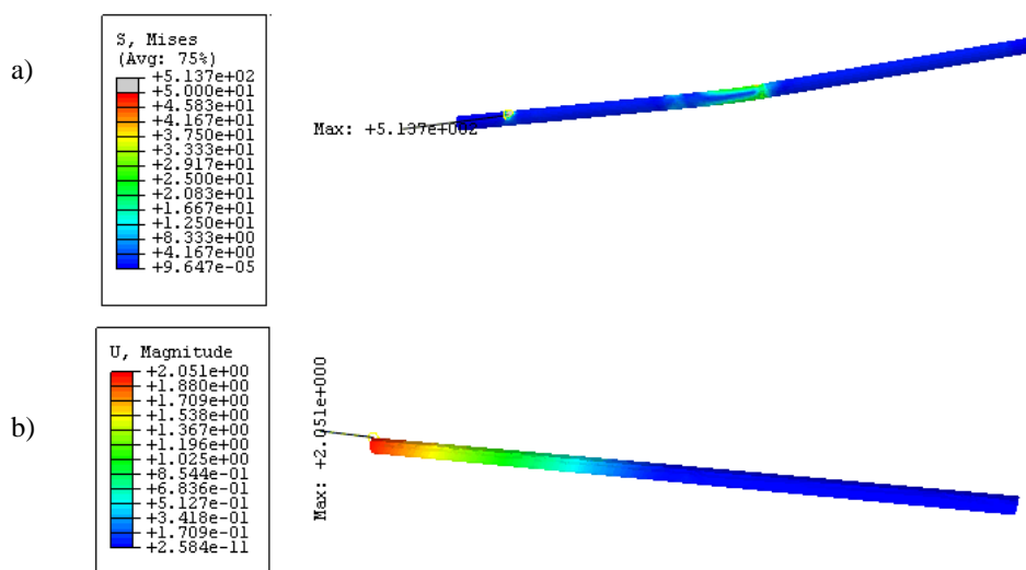
Slika 87. Model 3: raspodjela a) von Mises napreznja na koncu; b) pomaka na koncu
