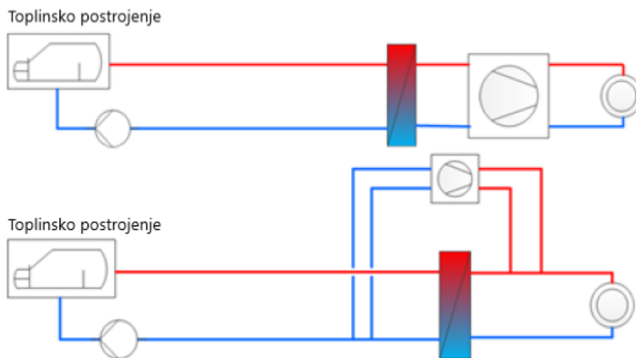
Slika 12. Integracija dizalice topline s unutarnjim izvorom za povećanje temperature sekundarne mreže [26]
