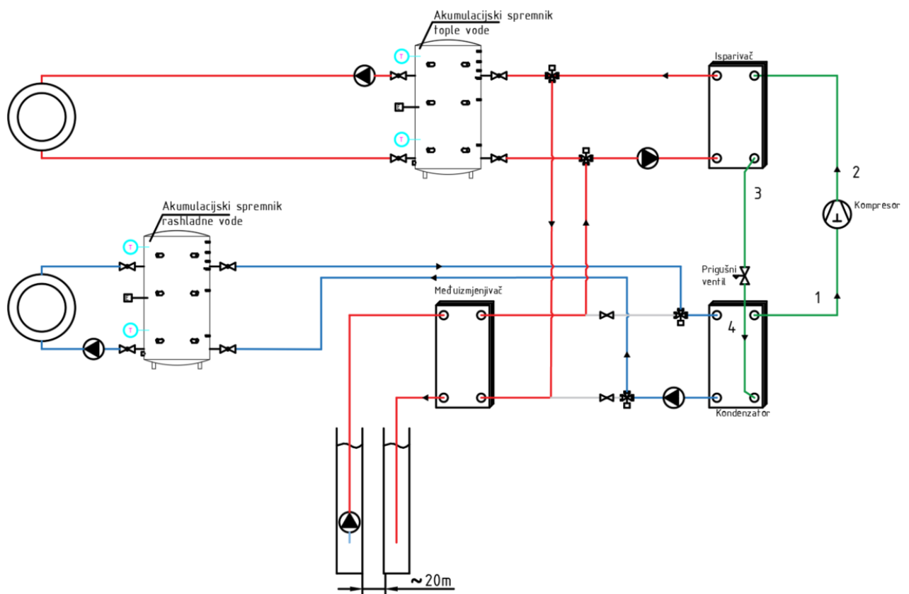
Slika 26. Shema jednostupanjske dizalice topline u režimu hlađenja
