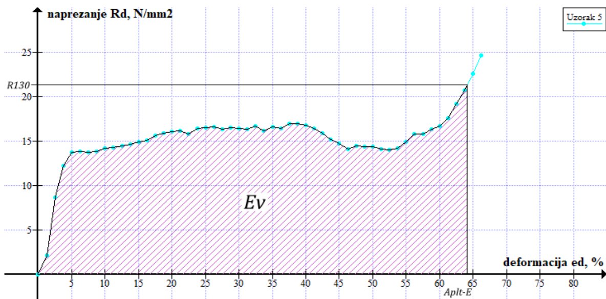
Slika 6.3.15 Dijagram naprezanje – deformacija, uzorak 5
