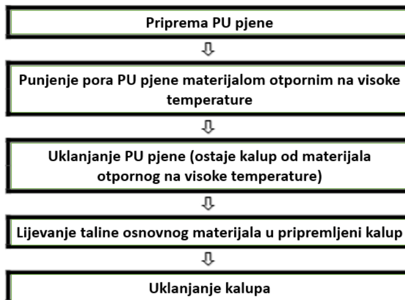
Slika 20. Faze preciznog lijevanja metalnih pjena [6]
