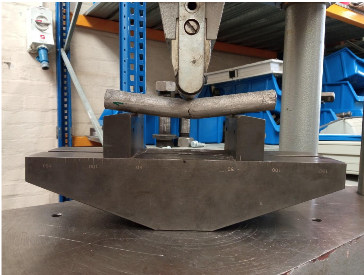
Slika 42. Naprava za ispitivanje savijanjem u tri točke
