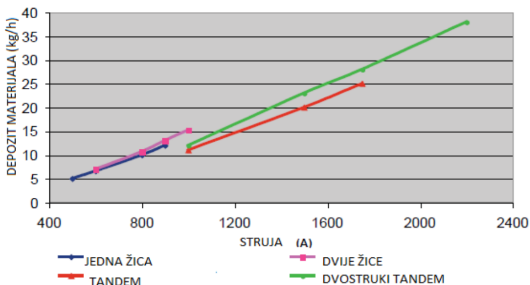
Slika 25. Usporedba produktivnosti inačica EPP zavarivanja [16]
