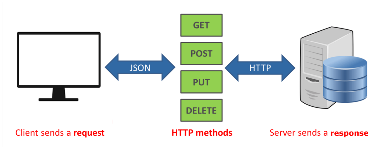
Slika 6. REST API[6]
