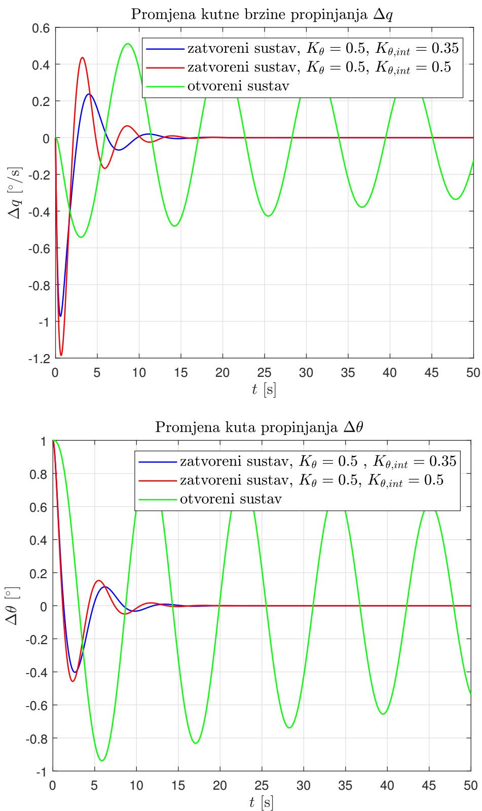
Slika 8.2: Prikaz promjene q i \theta otvorenog i zatvorenog sustava upravljanja stavom za V = 20.26 m/s, m = 55.26 kg
