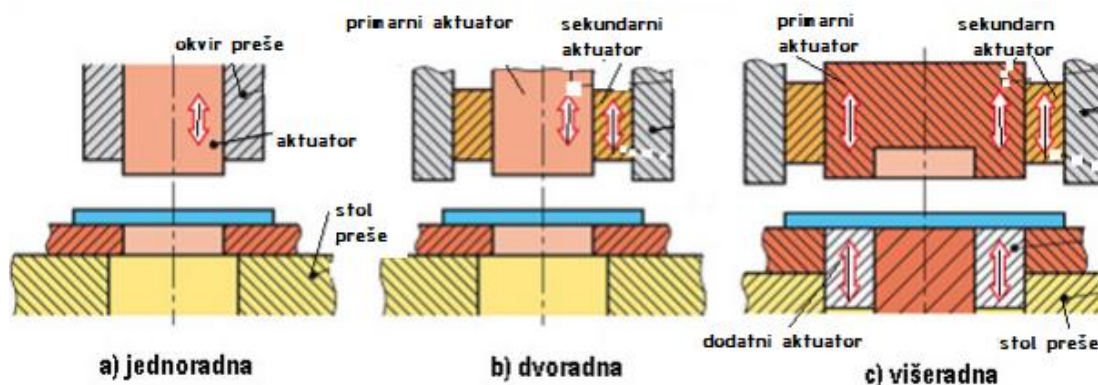
Slika 23. Podjela preša prema načinu rada [6]
