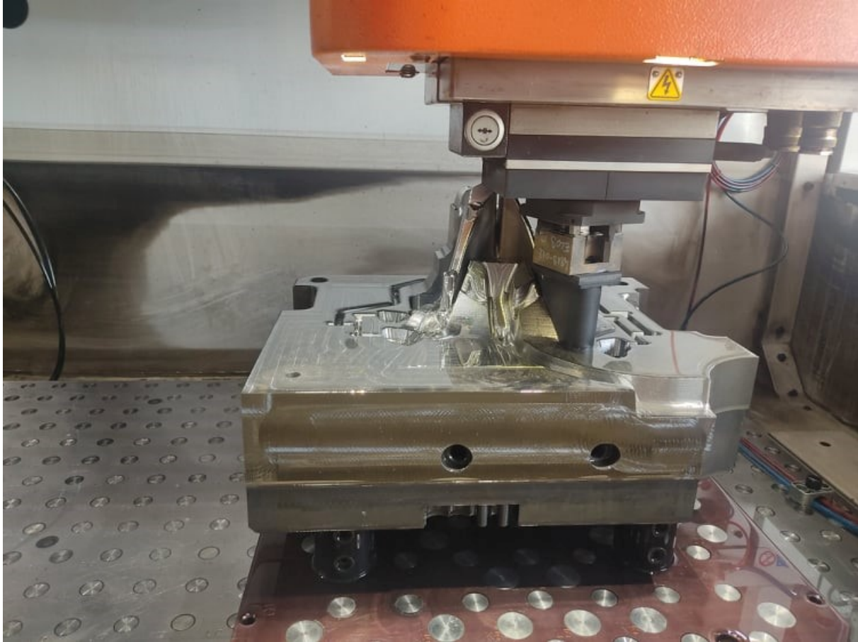
Slika 56. Izgled kalupnog uloška bez dielektrične tekućine
