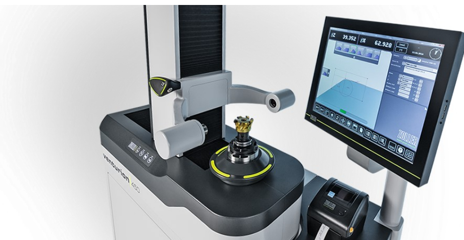
Slika 36. Uređaj za prednamještanje alata Zoller
