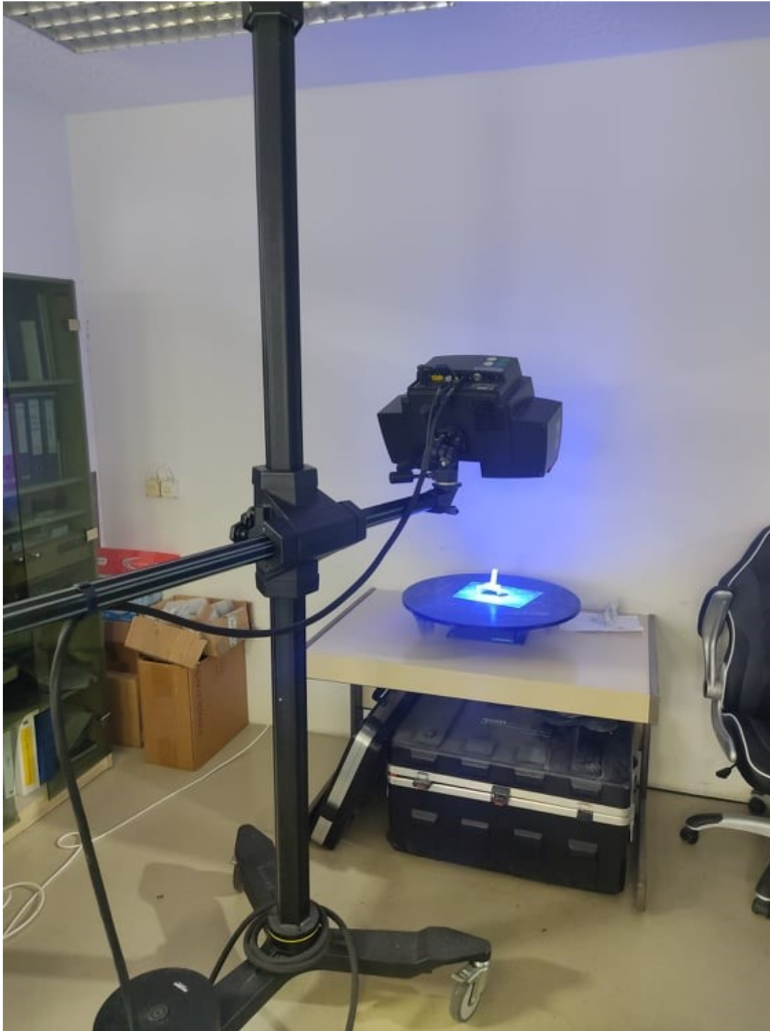
Slika 26. ATOS Triple Scan i plavo svjetlo
