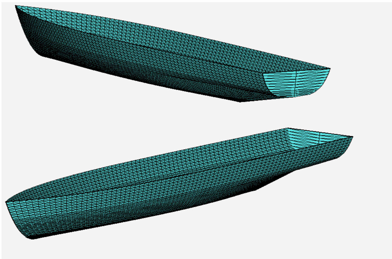
Slika 7. Triangularizirana analitička parametarska forma broda
