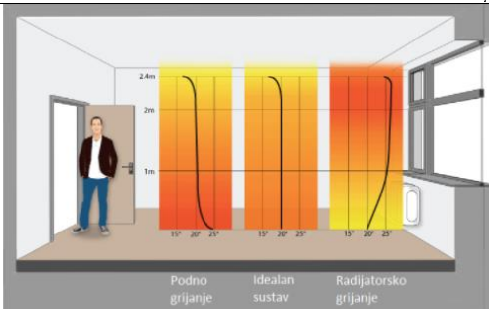
Slika 8. Distribucija topline kod podnog grijanja[7]
