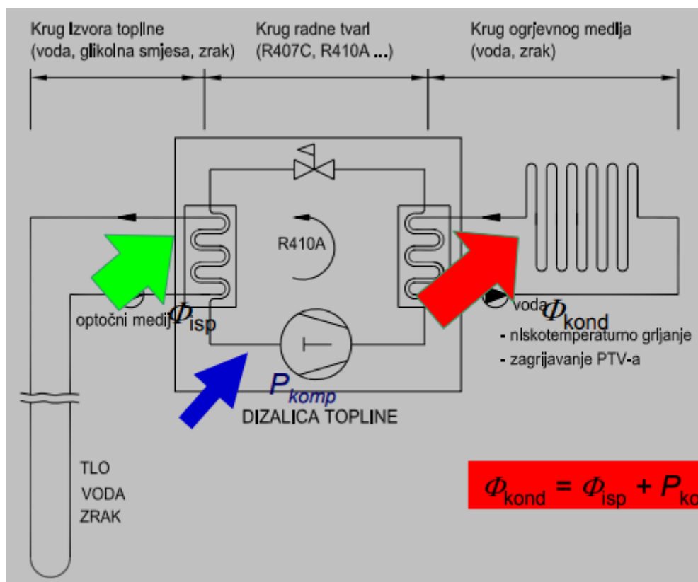
Slika 7. Shematski prikaz dizalice topline[5]
