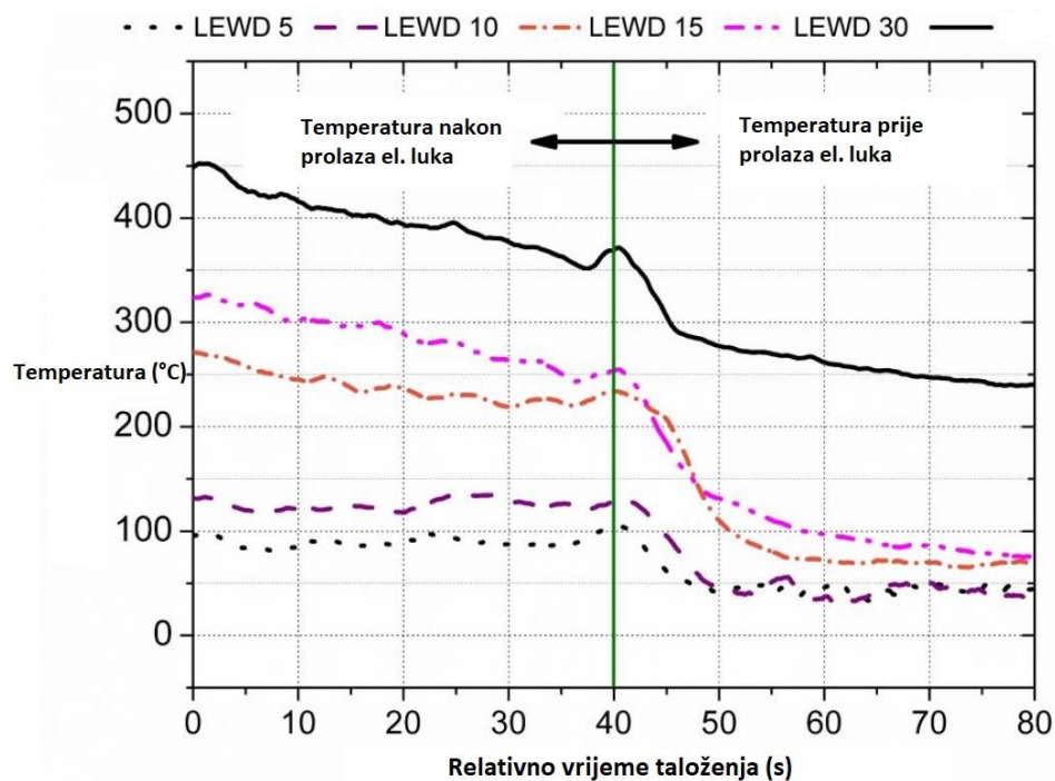
Slika 21. Utjecaj LEWD-a na međuprolaznu temperaturu [7]
