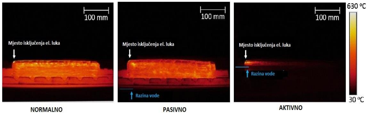
Slika 8. Termogrami uhvaćeni tik nakon završetka taloženja [9]
