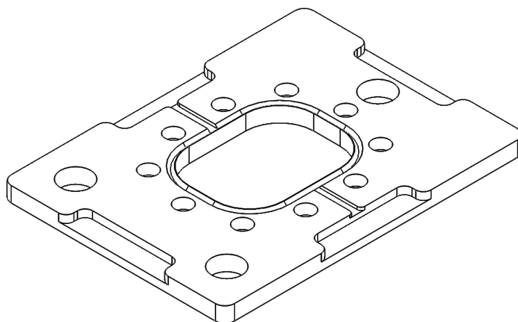
Slika 7.9. Srednja ploča kalupa za dobivanje kalupne šupljine (obruč)
